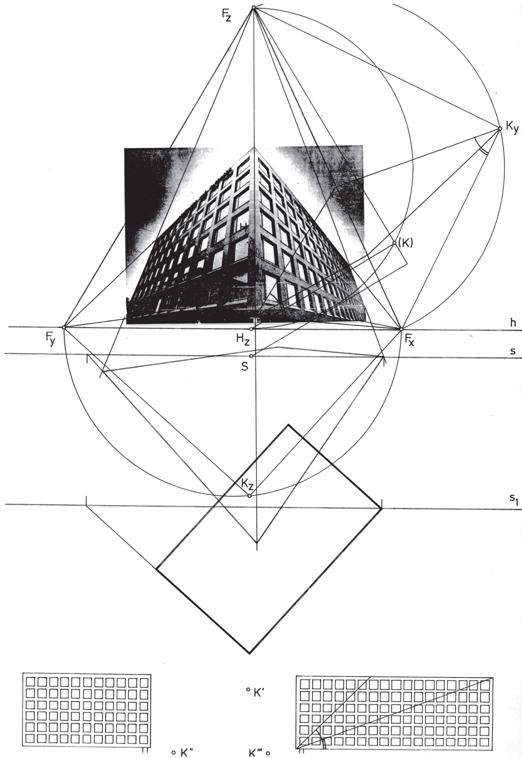
Kuva 4.4: Rekonstruktio vinosta perspektiivikuvasta (Helsingin Sähkötalo)
